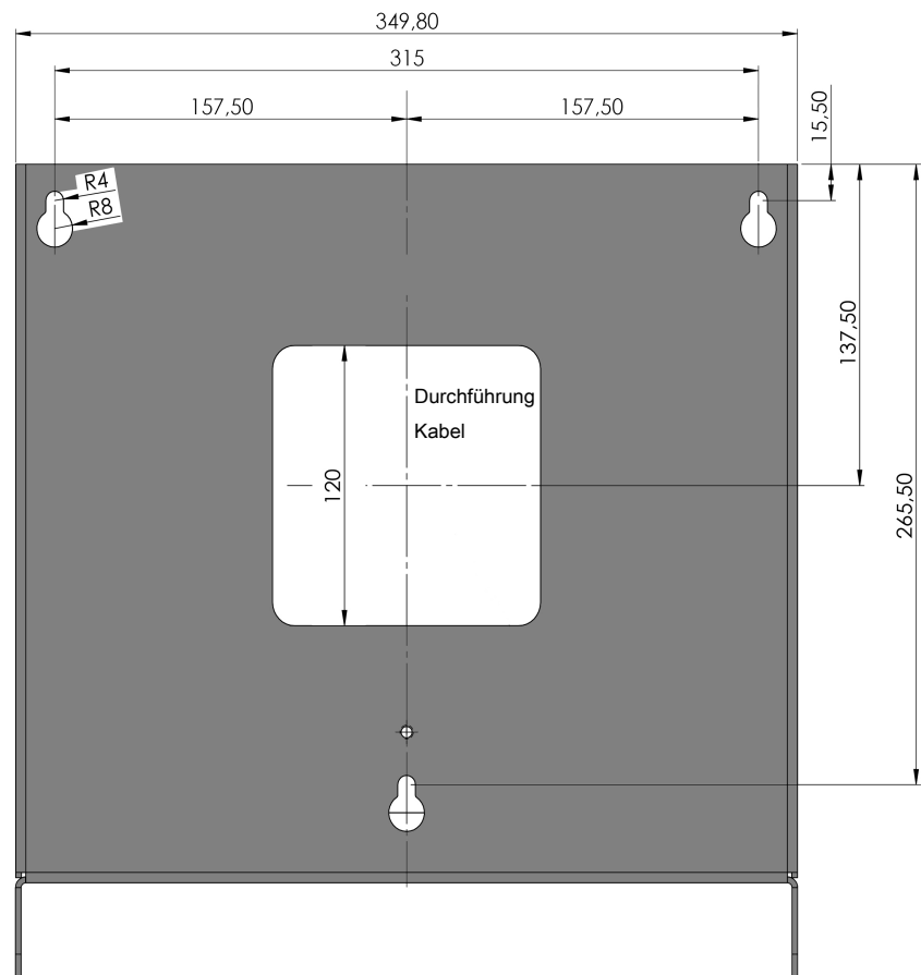
Abb. 2: Rückseite vom Geschossfang
