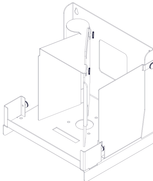
Abb. 1: Geschossfang Luftdruck
