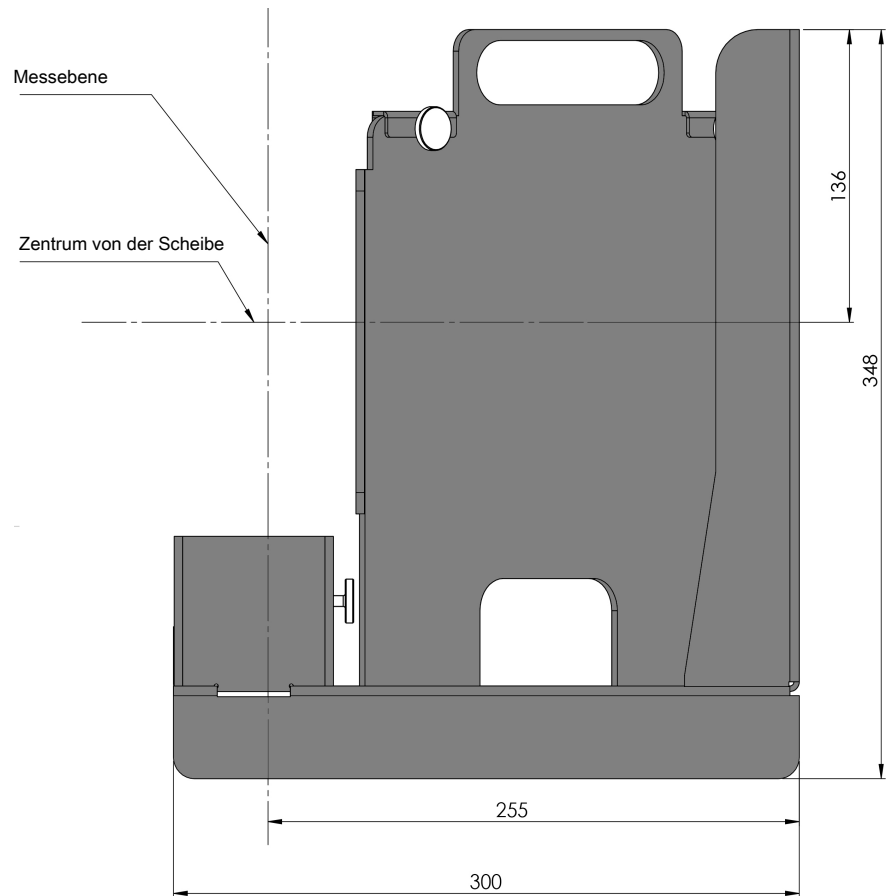
Abb. 3: Seite vom Geschossfang
